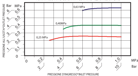
CARATTERISTICHE DI REGOLAZIONE*REGULATION FEATURES PORTATA COSTANTE*CONSTANT FLOW RATE=12,5 dm 3 /s(750 NI/min)
